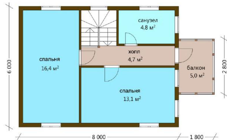
План 2 этажа
