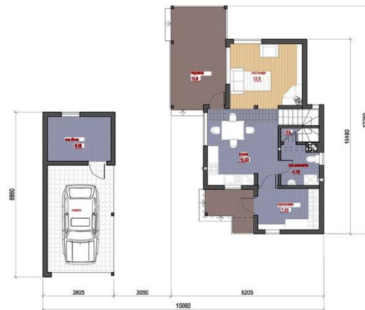
План 1 этажа
